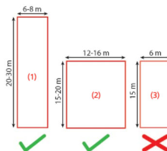
Illustration des formes parcellaires souhaitables (longueurs données à titre d'exemples) (schéma Géométrie)
